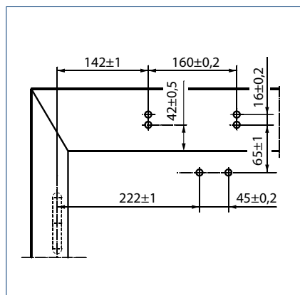
Anschlagsmaße Rechtstür
