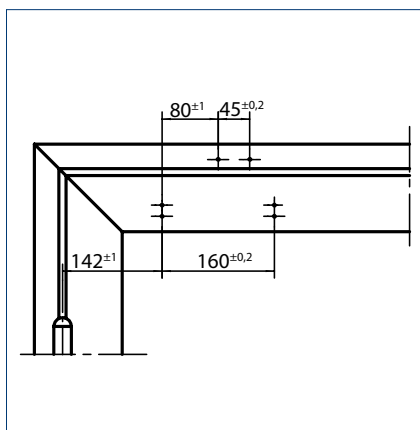
Anschlagmaße Linkstür
