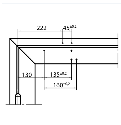
Anschlagmaße Linkstür
