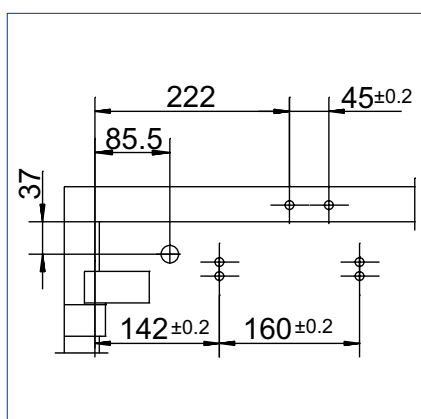
Anschlagmaße Linkstür
