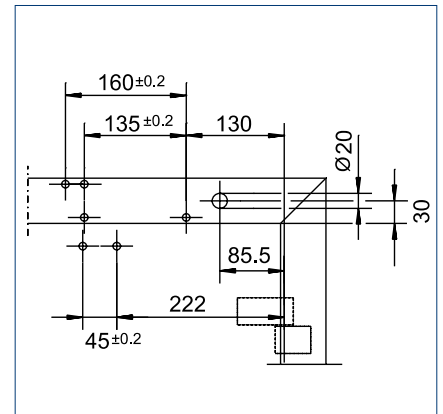
Anschlagsmaße Linkstür
