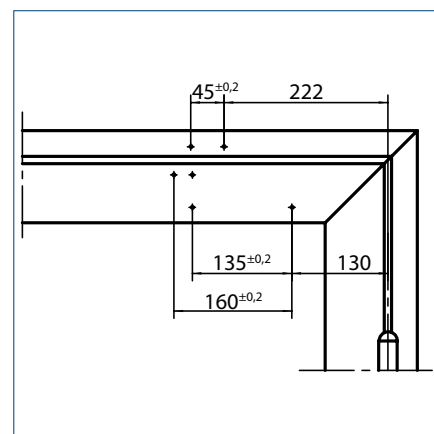
Anschlagmaße Rechtstür
