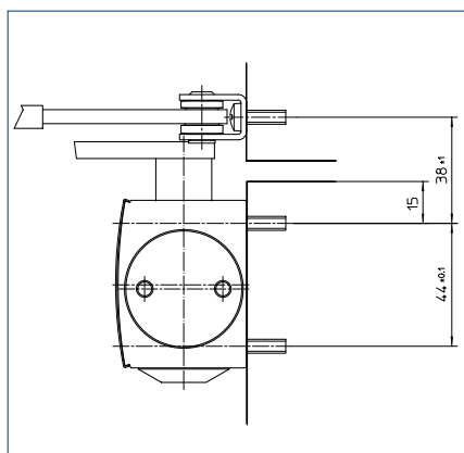
Schnitt = Direktmontage
