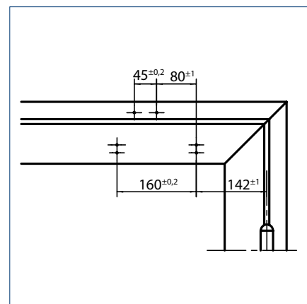
Anschlagmaße Rechtstür
