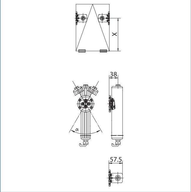
Drehkonsole
