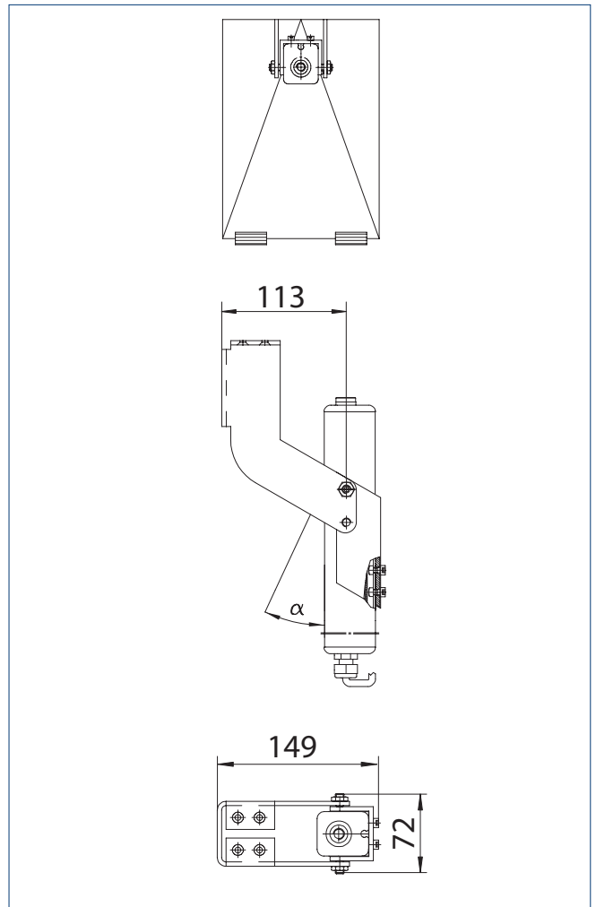
Konsole EINWÄRTS
