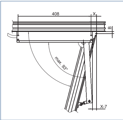
Draufsicht
